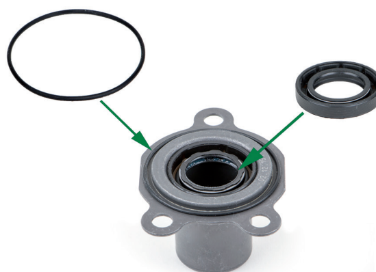
Направляющая втулка с предустановленным уплотнительным кольцом и уплотнением вала
