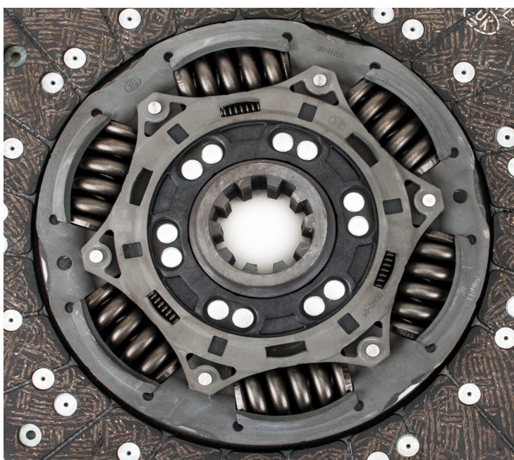
Шесть пружинных демпферов с демпфером первой ступени
