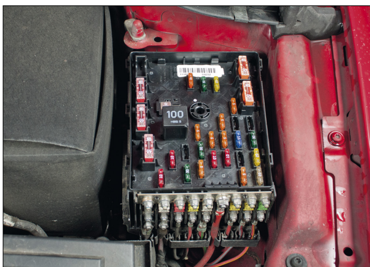
Рисунок 1: Предохранитель системы мехатроники, как правило, расположен в блоке предохранителей, находящемся в моторном отсеке
