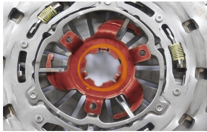
Рис. 4: Блокирующий элемент
