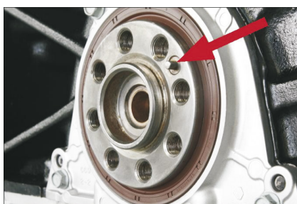
Рис.1: Установочный штифт коленвала
