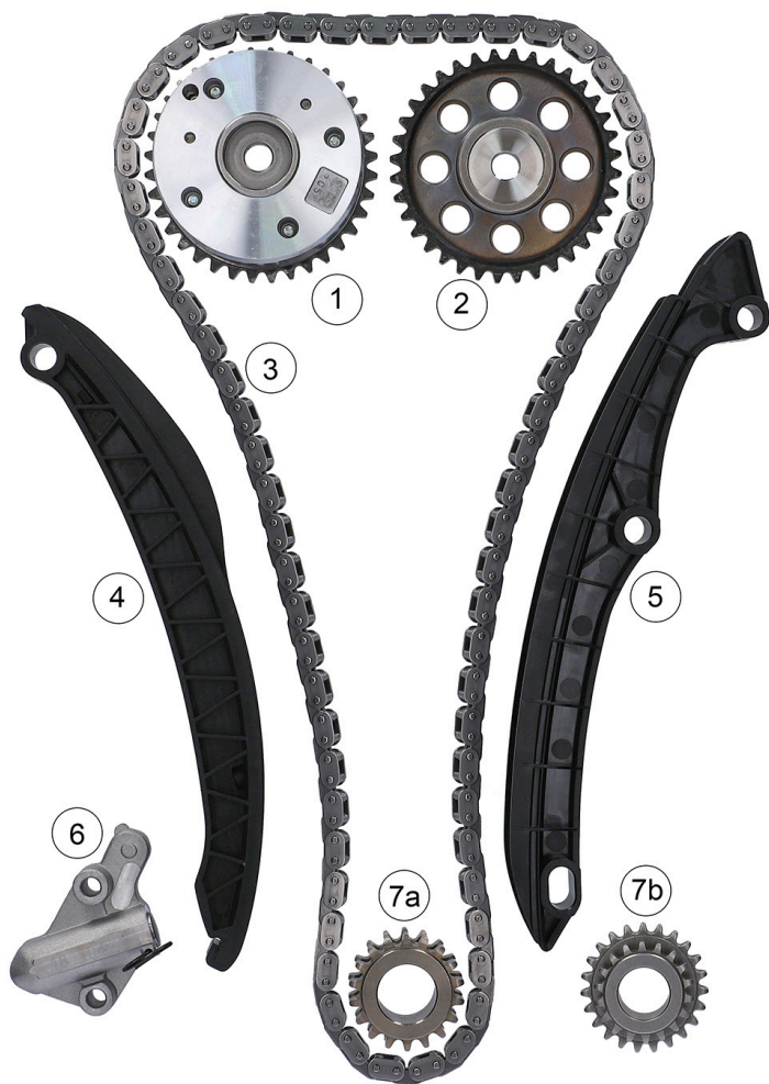
Рисунок 1: 559 0154 30/559 0154 31 – компоненты комплекта привода ГРМ
