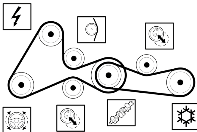
Рис. 1: Ременной привод для двигателей с номерами до 0113089 с натяжным роликом
