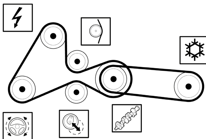
Рис. 2: Ременной привод для двигателей с номерами от 0113090 с эластичным ремнем
