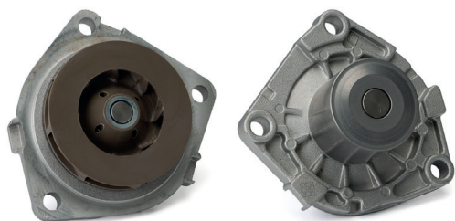
Рисунок 1: 538 0310 10 – насос охлаждения со стандартным подшипником.
