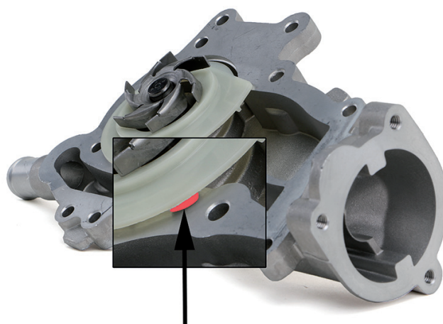
Рис. 2: Деформация пластикового корпуса ввиду нанесения чрезмерного количества герметика
