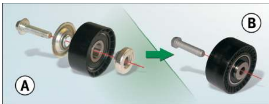
Обводной ролик 532 0433 10, предыдущая конструкция (A) и новая (B)
