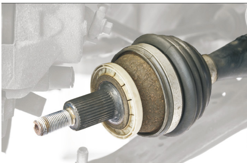
Рис. 1: Сальники могут отличаться по конструкции и цвету!
